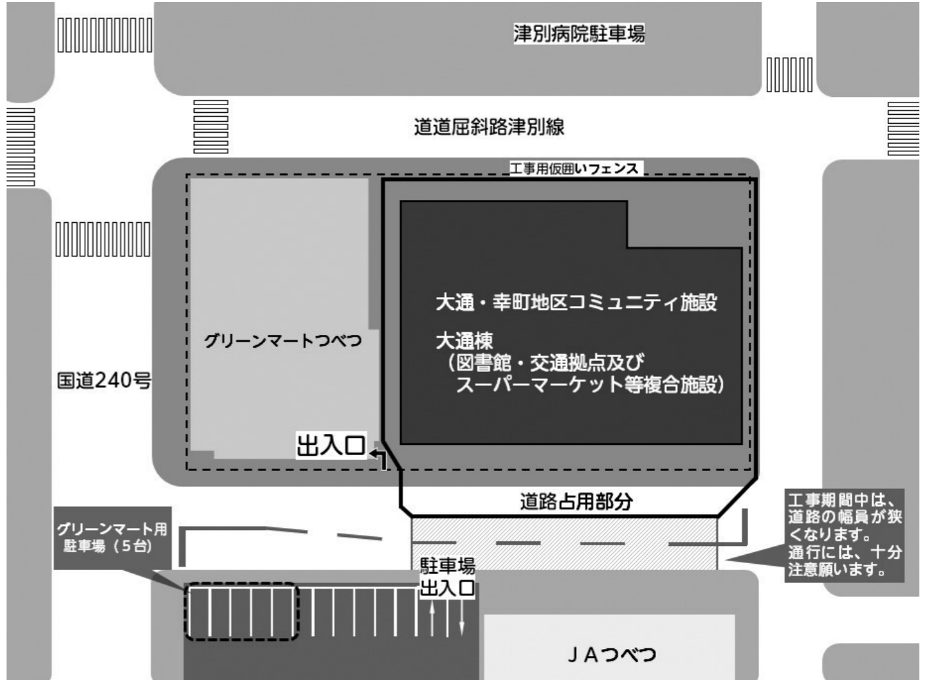
まちなか再生事業 大通・幸町地区コミュニティ施設「大通棟」配置図および仮設計画
