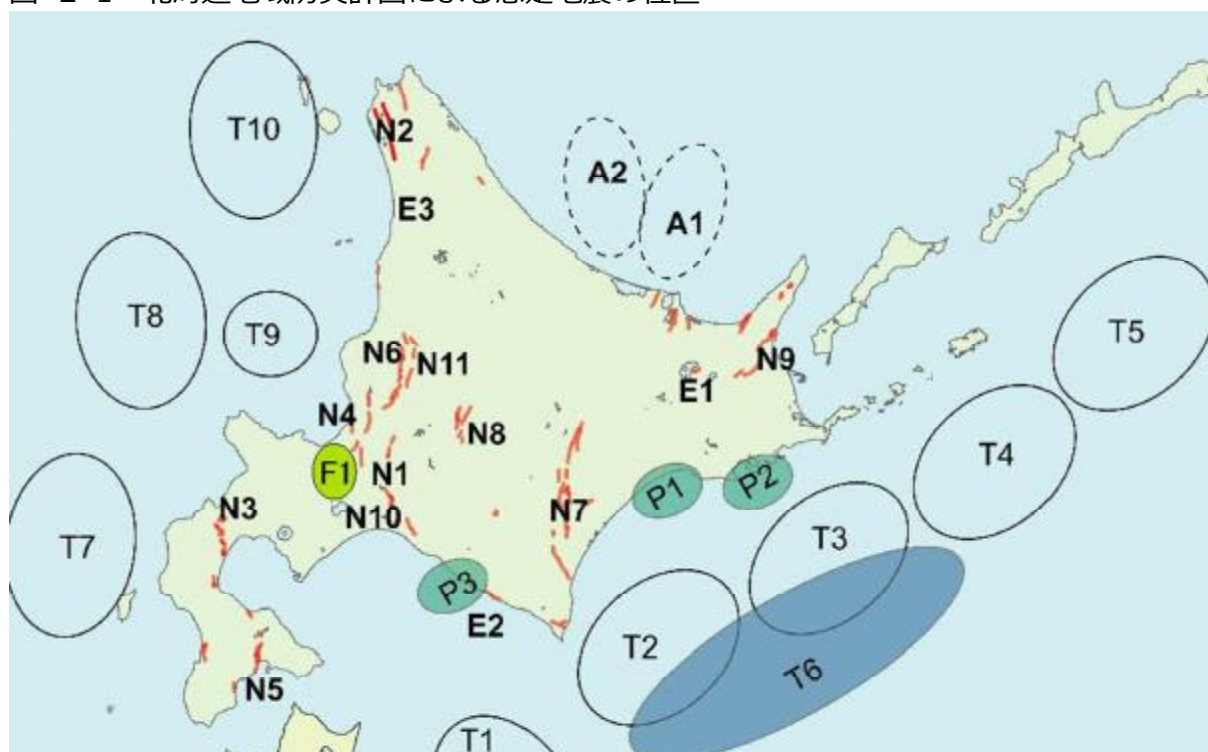
図 2-1 北海道地域防災計画による想定地震の位置
