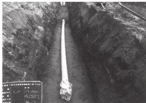
H28管路掘削状況（上）管布設エポリエチレン管（下）
